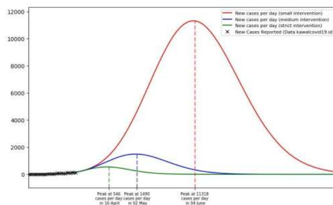
Gambar 7. Grafik Perbedaan Dari Tiga Skenario Pembatasan Kontak Fisik
