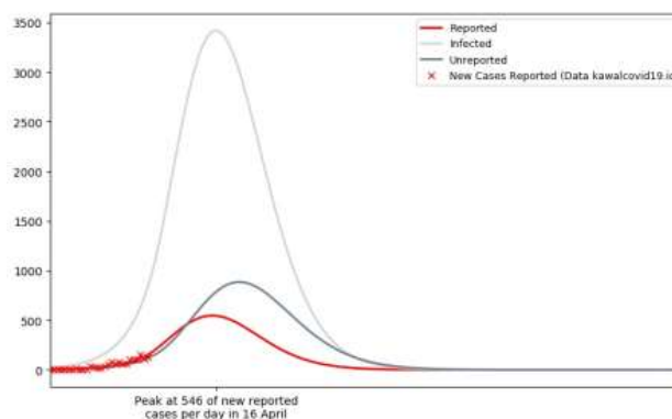
Gambar 6. Grafik Pertumbuhan Kasus Positif Covid-19 dengan Model SIRU
